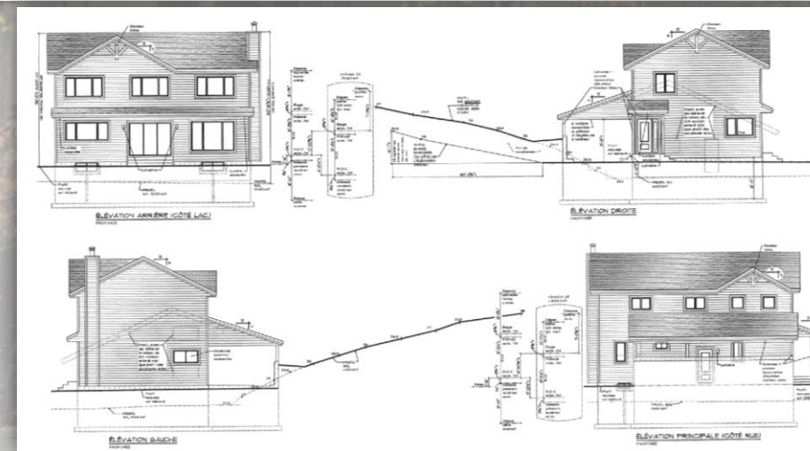
ÉLÉVATION ARRIÈRE PROPOSÉE VUE DU LAC
