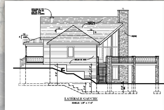
Bâtiment principal projeté
