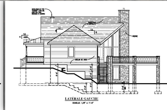
Bâtiment principal projeté
