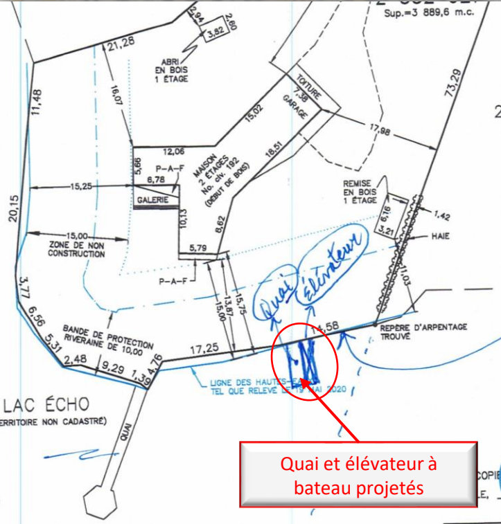
Implantation projetée
