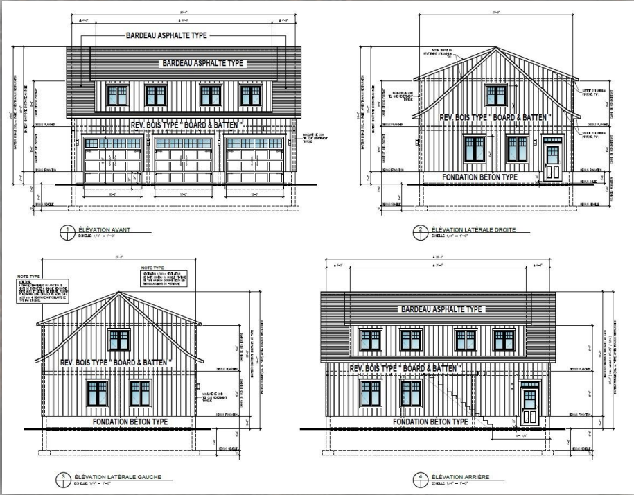
Garage projeté
