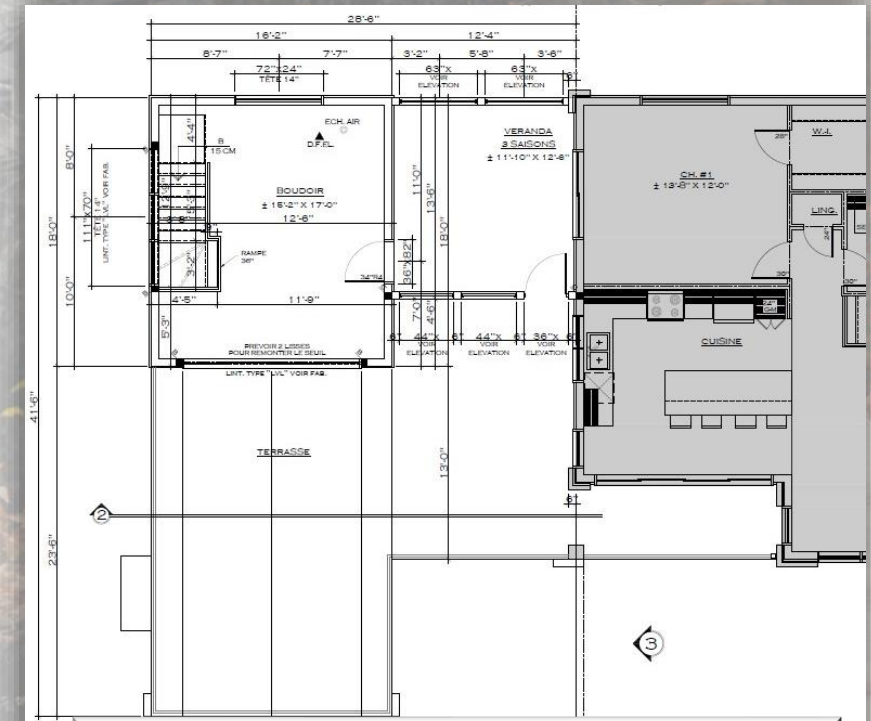
Plan de l'étage – Ajout de 288 pi 2 , soit 14,9% de 1939 pi 2 (situation conforme)
